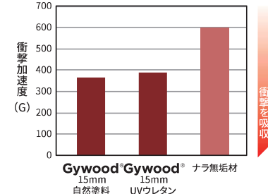
Gywood® 衝撃吸収試験
